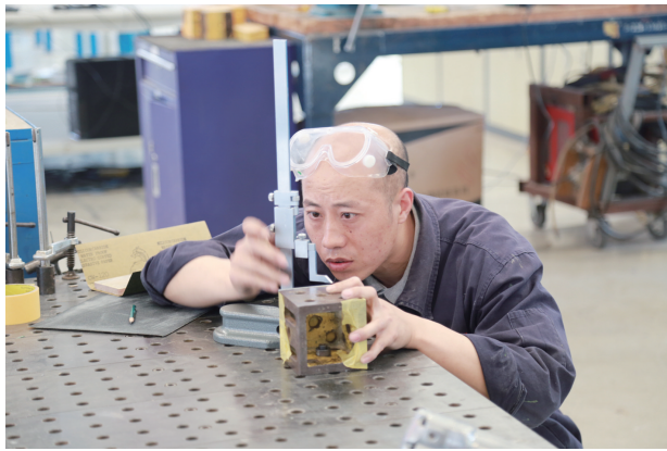
国产大飞机分舱板型材装配产线。
